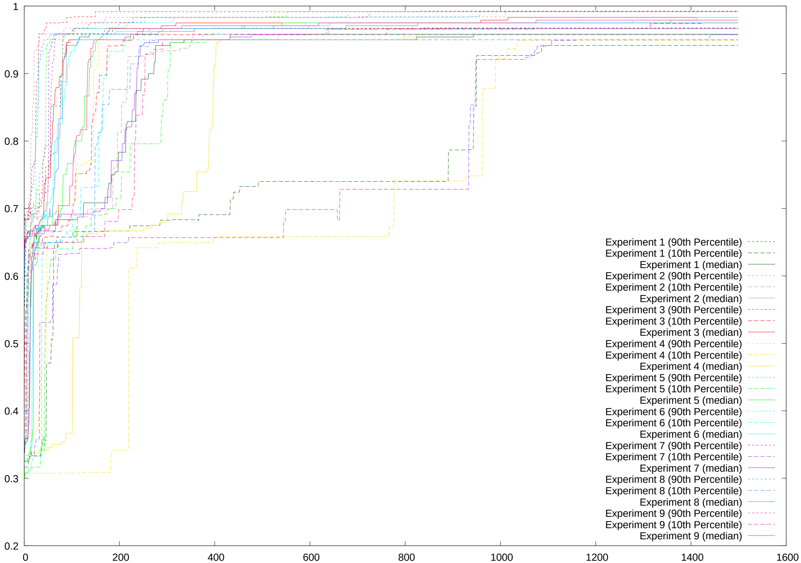
Accuracy auf den Trainingsdaten über die Zeit (Datensatz Iris, Trainiert auf balancierter Accuracy)
